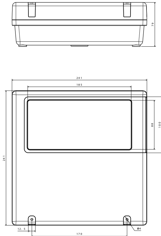
dimensiones generales.
