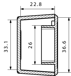
Corte B-B. Escala: 1:1
