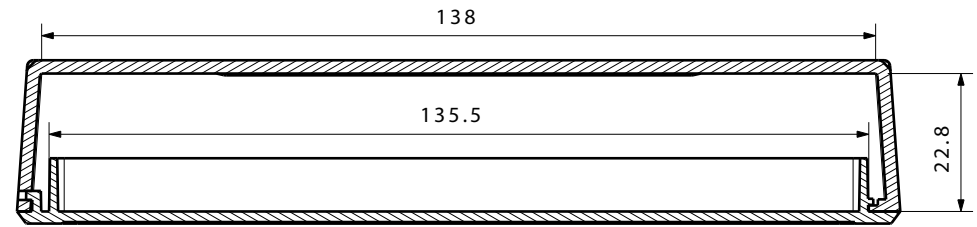
Corte A-A. Escala: 1:1
